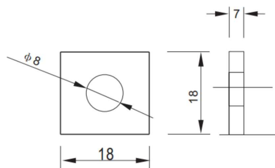
M6 BOLT&NUT
